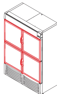
ENSAMBLE DE PUERTA
