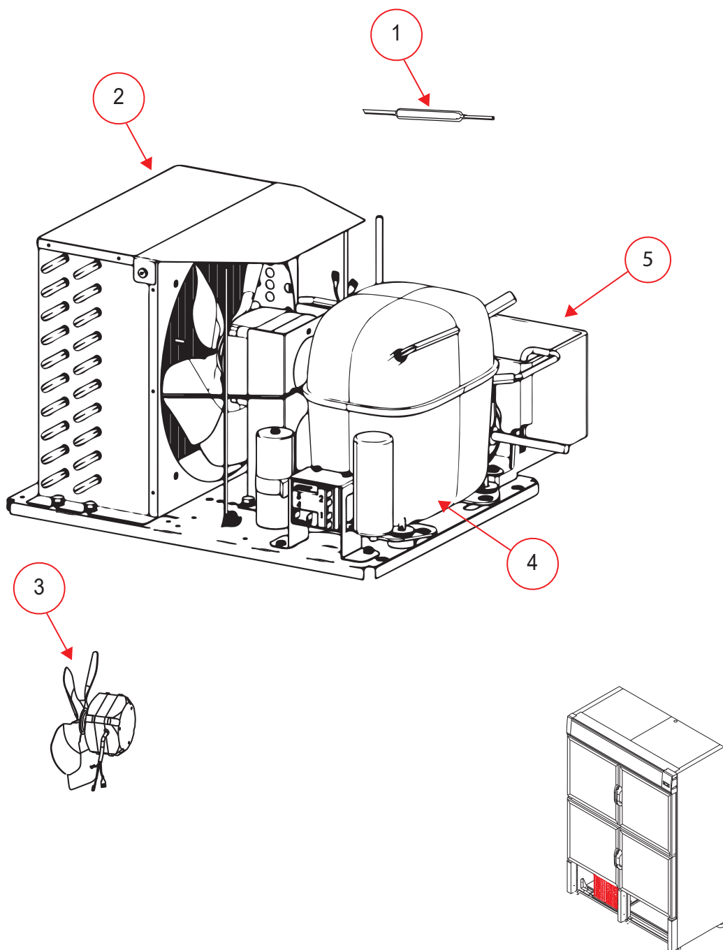
ENSAMBLE CONDENSADOR
