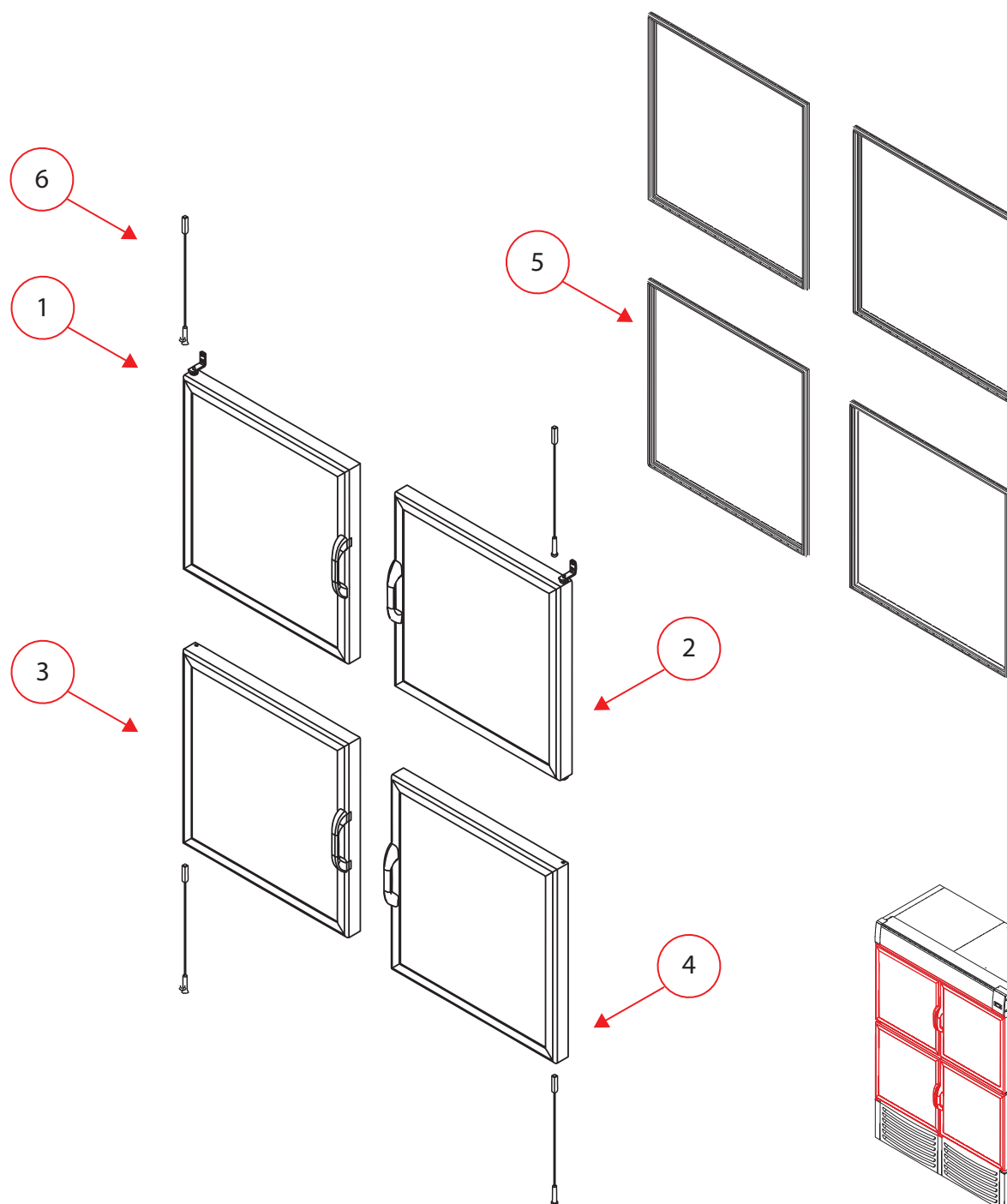
ENSAMBLE DE PUERTA
