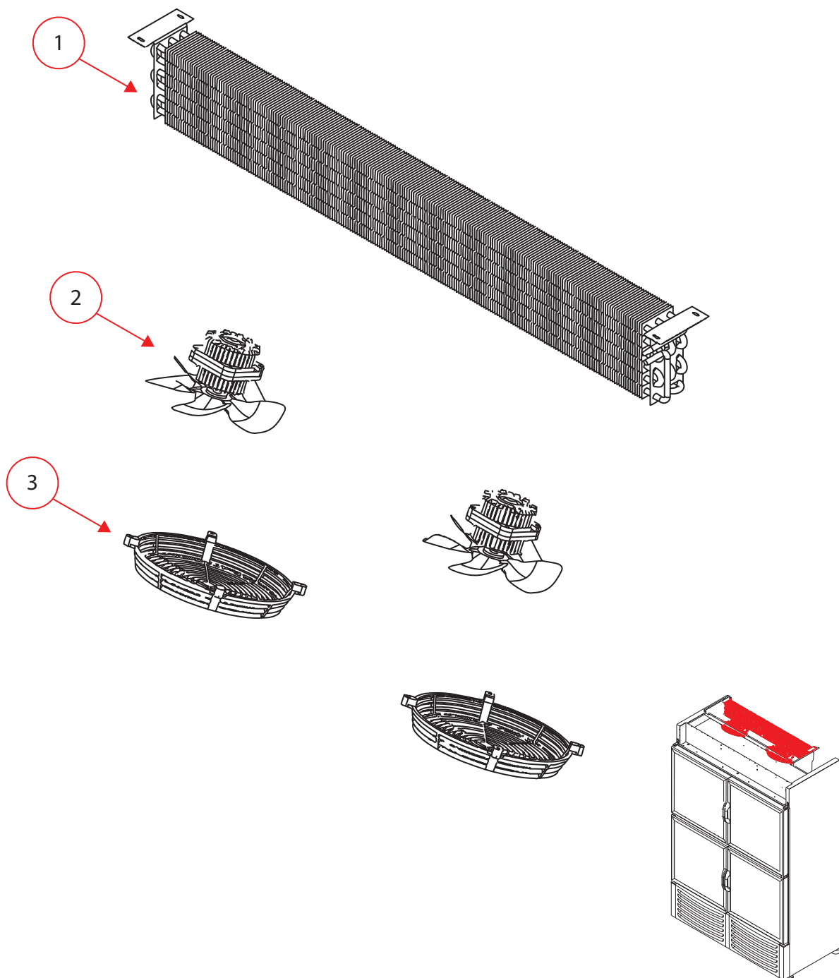
ENSAMBLE EVAPORADOR
